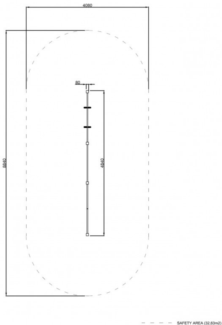
Rys. 1. Wymiary urządzenia i strefy bezpieczeństwa
